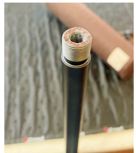
Korrosionsschaden am Laufgewinde
